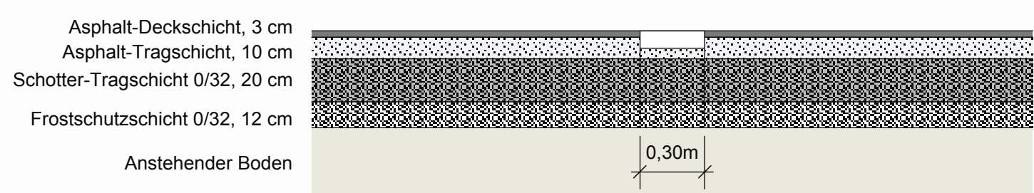
Schnitt B-B: Asphaltbetonweg mit Betonrillenplatten-Streifen, 1 : 25
