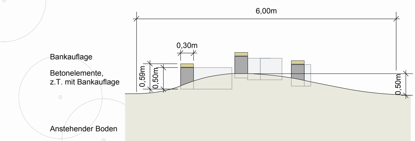
Schnitt E-E: Hügel mit Betonsitzelementen 0,30 x 0,50 x 2-3m, 1 : 50
