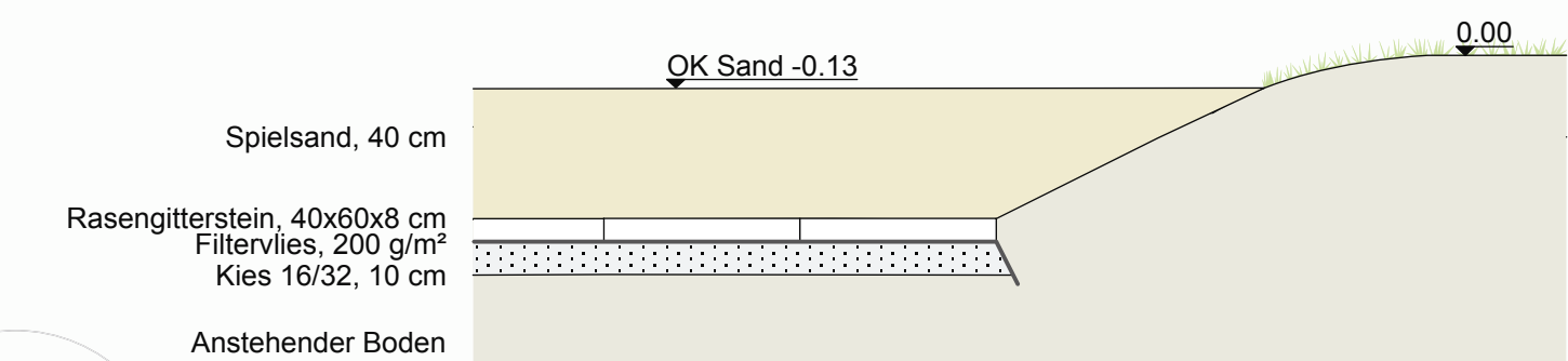
Schnitt D-D: Übergang Rasen - Sandfläche, 1 : 25
