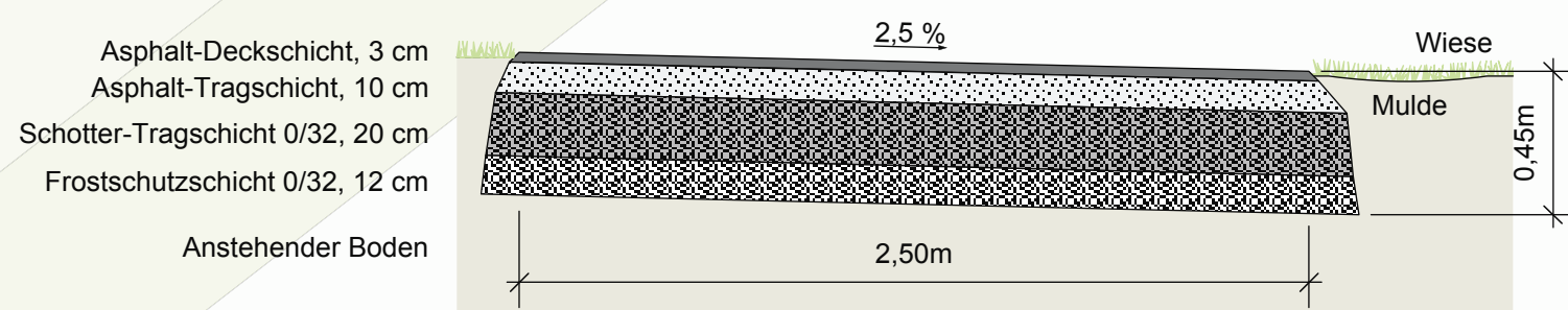
Schnitt A-A: Asphaltbetonweg Gesamtaufbau 0,45m, 1 : 25
