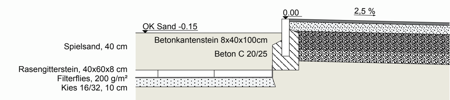
Schnitt C-C: Abgrenzung Asphaltweg - Sandfläche, 1 : 25
